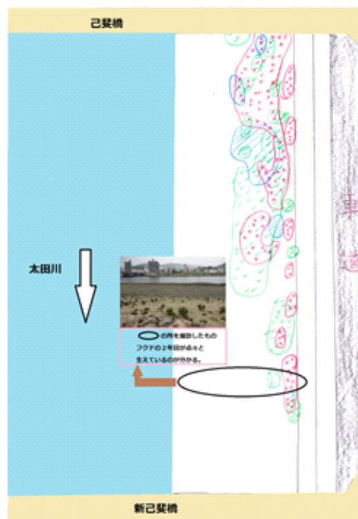
図21 己斐橋～新己斐橋 左岸の分布図 調査日:2013年4月5日
