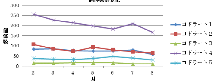
図 24 コドラート別のフクドの2年目の 個体数の変化
