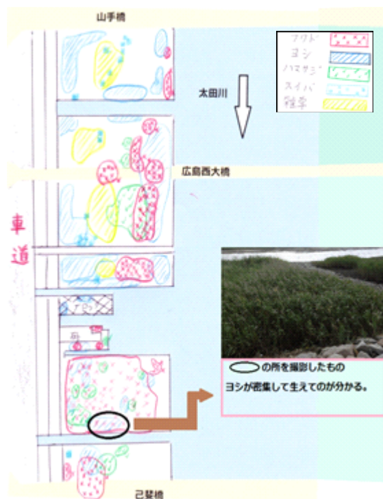
図18 山手橋～己斐橋 右岸の分布図 調査日:2013年3月7日
