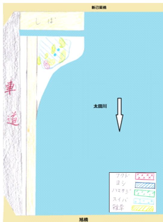
図22 新己斐橋～旭橋 右岸の分布図 調査日:2013年4月5日
