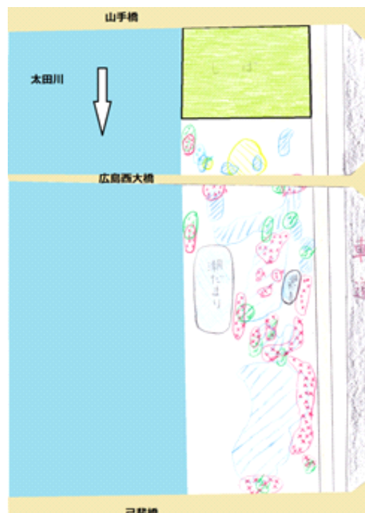
図19 山手橋～己斐橋 左岸の分布図 調査日:2013年3月30日, 4月5日
