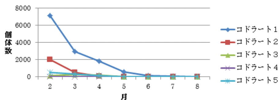
図 26 コドラート別のフクドの1年目の 個体数の変化
