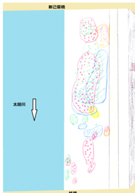
図23 新己斐橋～旭橋 左岸の分布図 調査日:2013年4月5日
