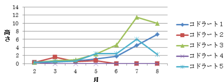
図 27 コドラート別のフクドの1年目の 中央個体の高さの変化
