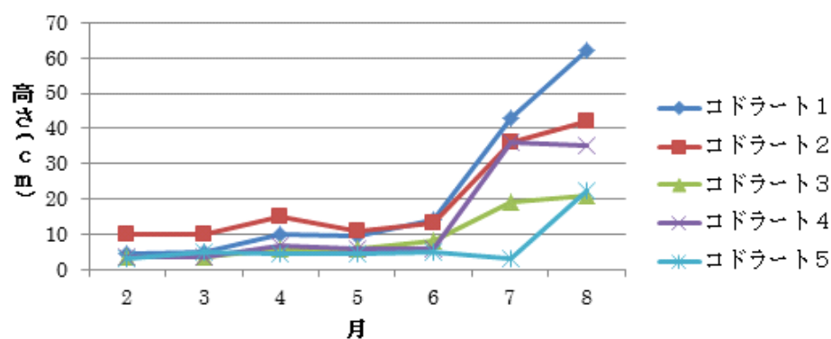
図 25 コドラート別のフクドの2年目の 中央個体の高さの変化
