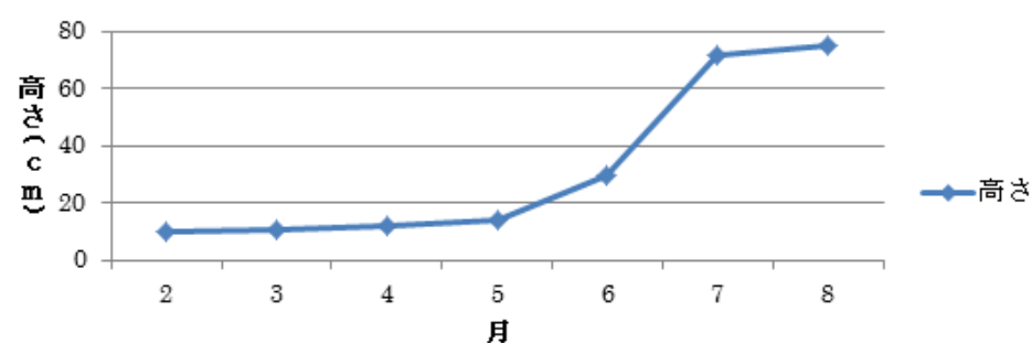
図 28 コドラート 1における ハマサジの2年目（1個体）の高さの変化
