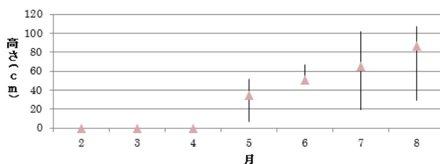
図 29 コドラート 3における ヨシの1年目の高さの変化
