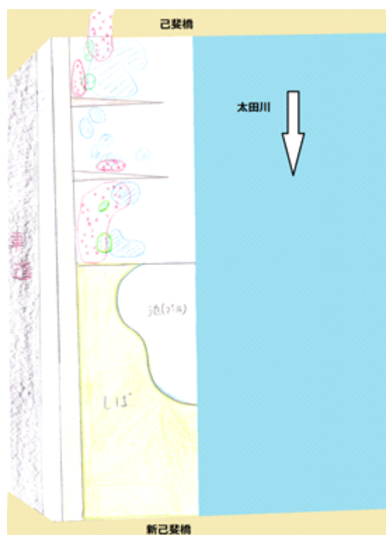
図20 己斐橋～新己斐橋 右岸の分布図 調査日:2013年3月30日
